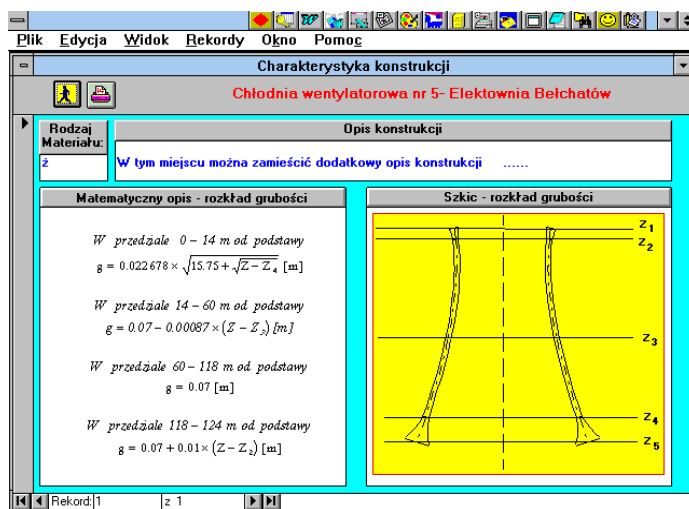
Rys 5. Przykład edycji danych o konstrukcji chłodni
