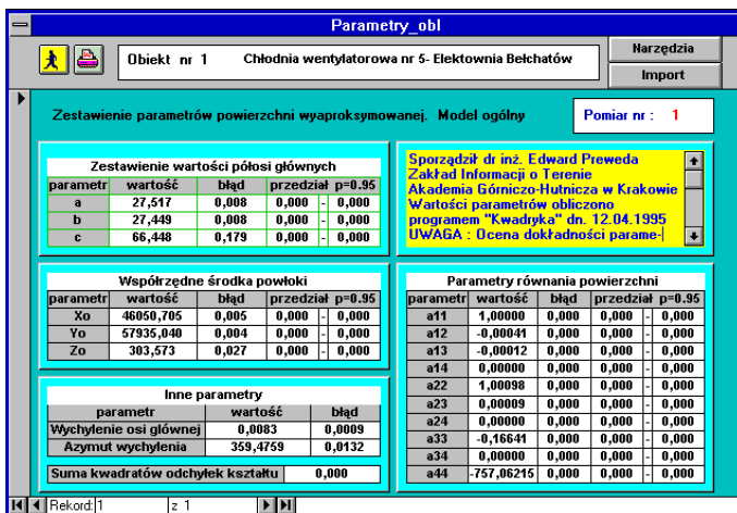
Rys. 7 Postać formularza służącego do wprowadzenia /importu estymowanych parametrów hiperboloidy jednopowłokowej
